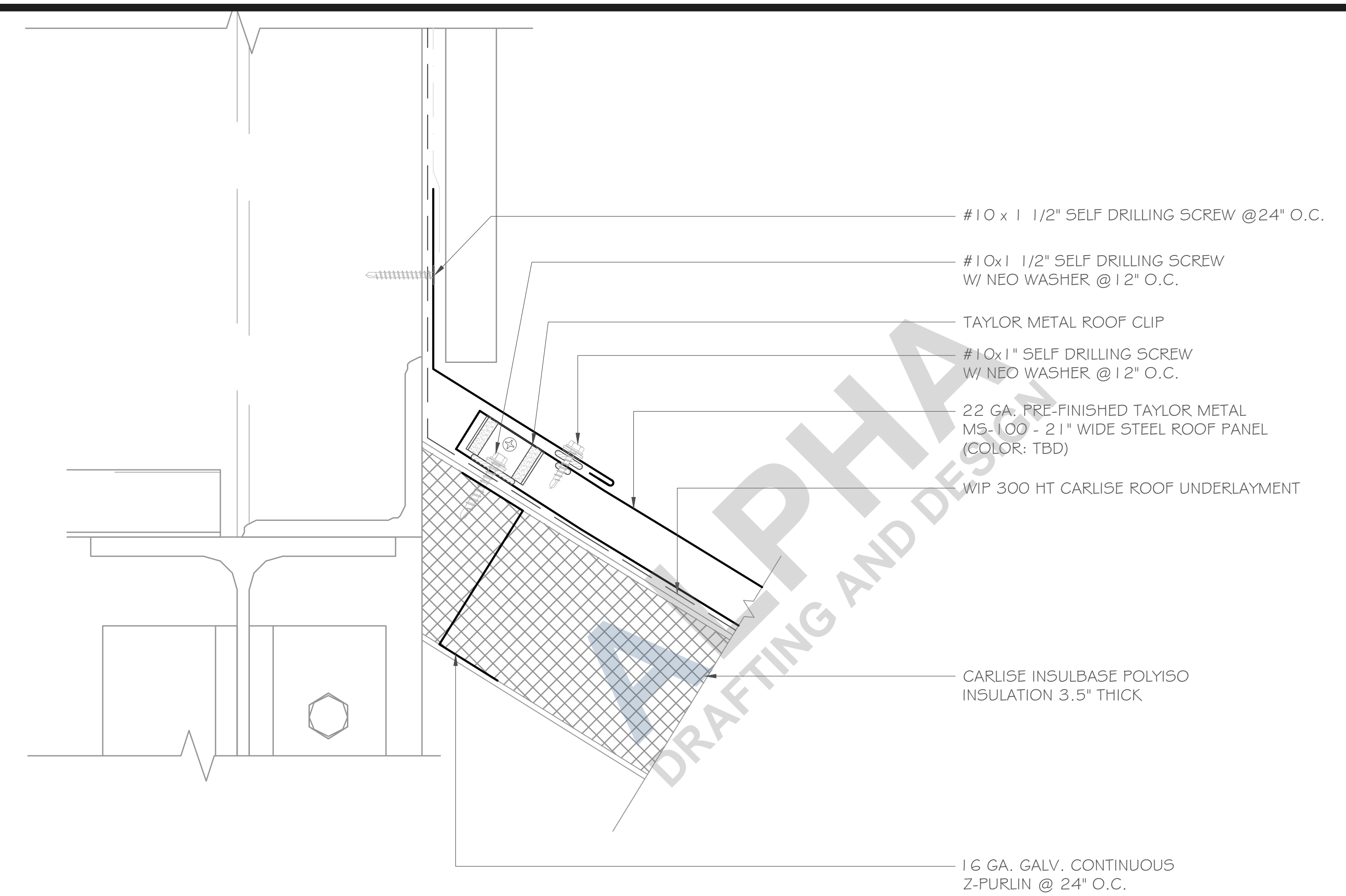
3 WALL DETAIL SCALE: 6"=1'-0" REF.: --
