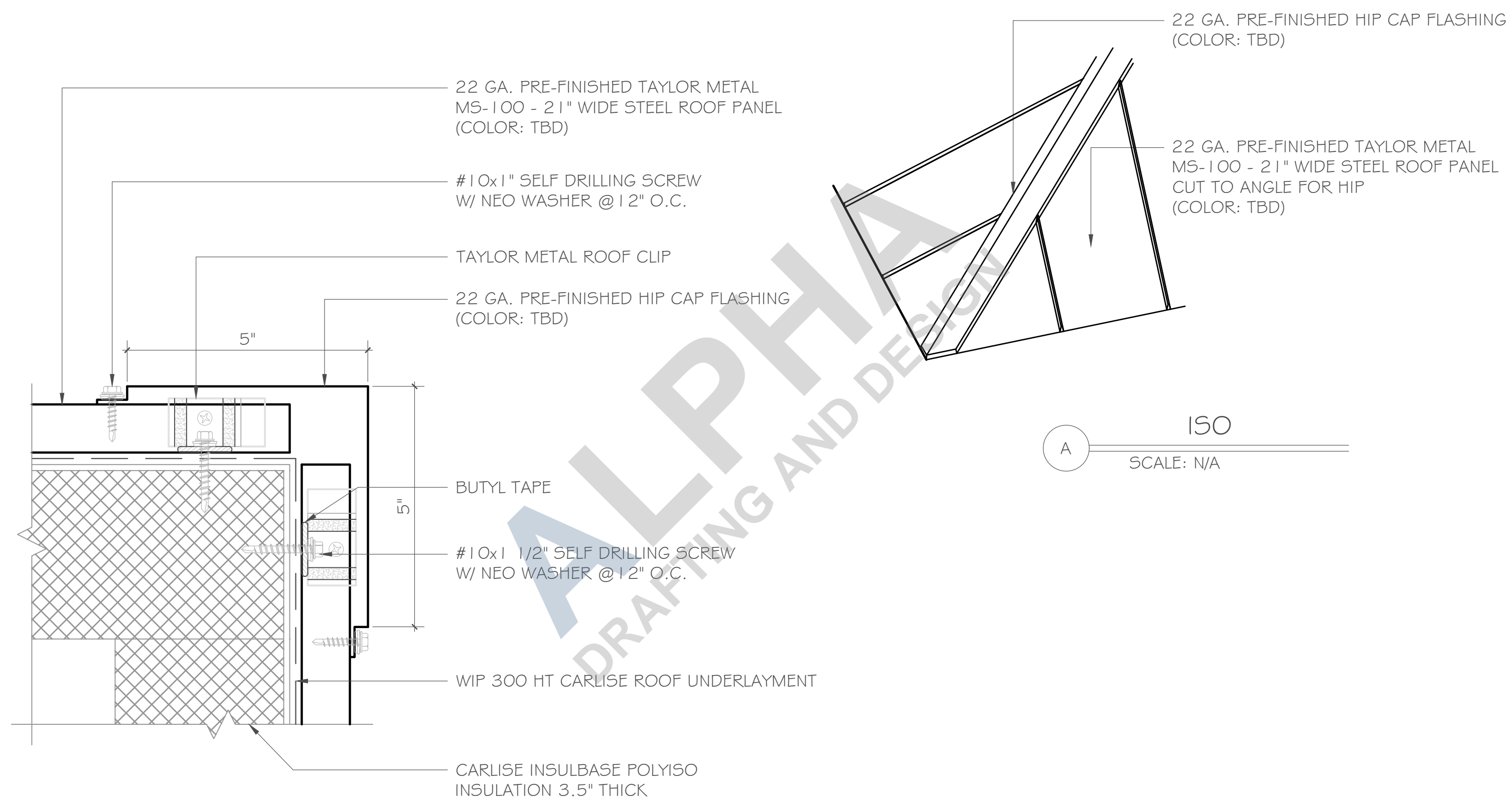
1 HIP DETAIL SCALE: 6"=1'-0" REF.: --
